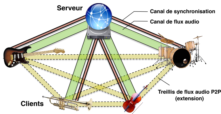
Fig. 1: Modélisation du client-serveur de jam session
